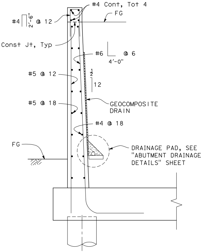
SECTION D-D
