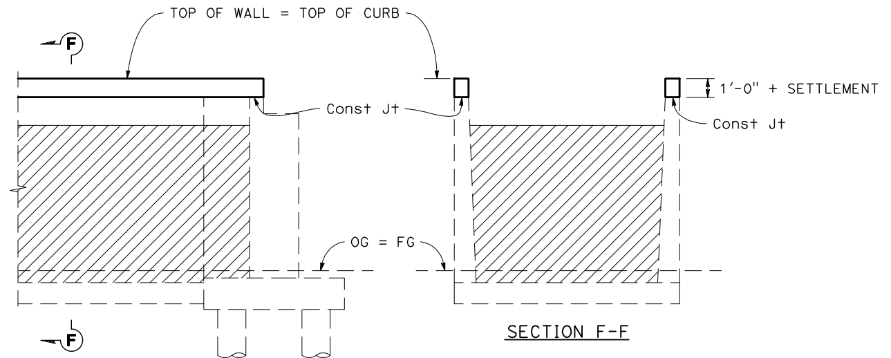
STEP 5
