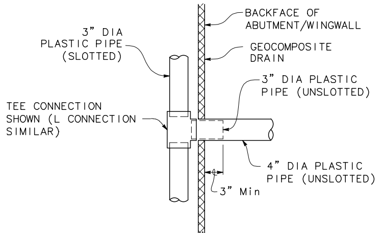
T-CONNECTION
